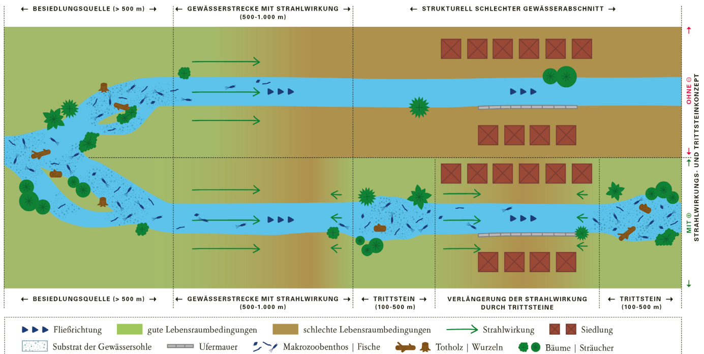
ABBILDUNG 1: Strahlwirkungs- und Trittsteinkonzept in der Landesstudie Gewässerökologie
